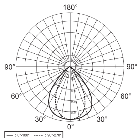
Distribución de Intensidad Luminosa [cd/KLm]
